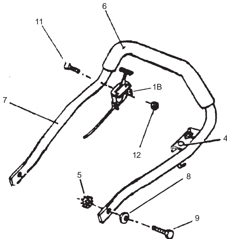
Fig. 2 Non-Clutch
